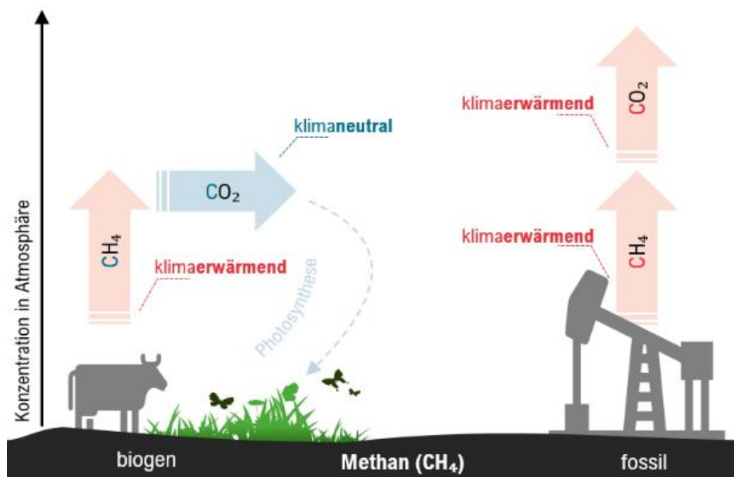
Abbildung 5: Klimawirkung von biogenem und fossilem Methan 1614
