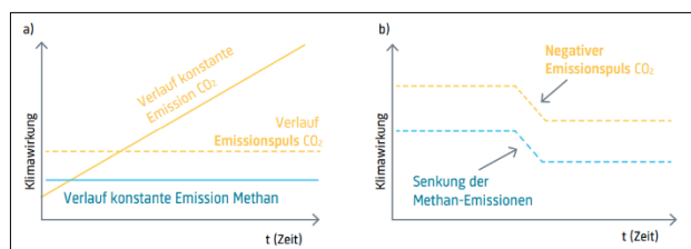
Abbildung 4: Vergleich der Klimawirkung von Emissionsverläufen der CO 2 - und Methanemissionen bei einer konstanten Emission (a) und einer Emissionsreduktion (b) 13
