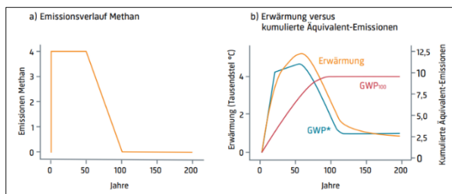
Abbildung 6: Der GWP* kann Zeitverläufe und entsprechend die Klimawirkung kontinuierlicher kurzlebiger Gase im Vergleich zum GWP 100 besser abbilden 13 .
